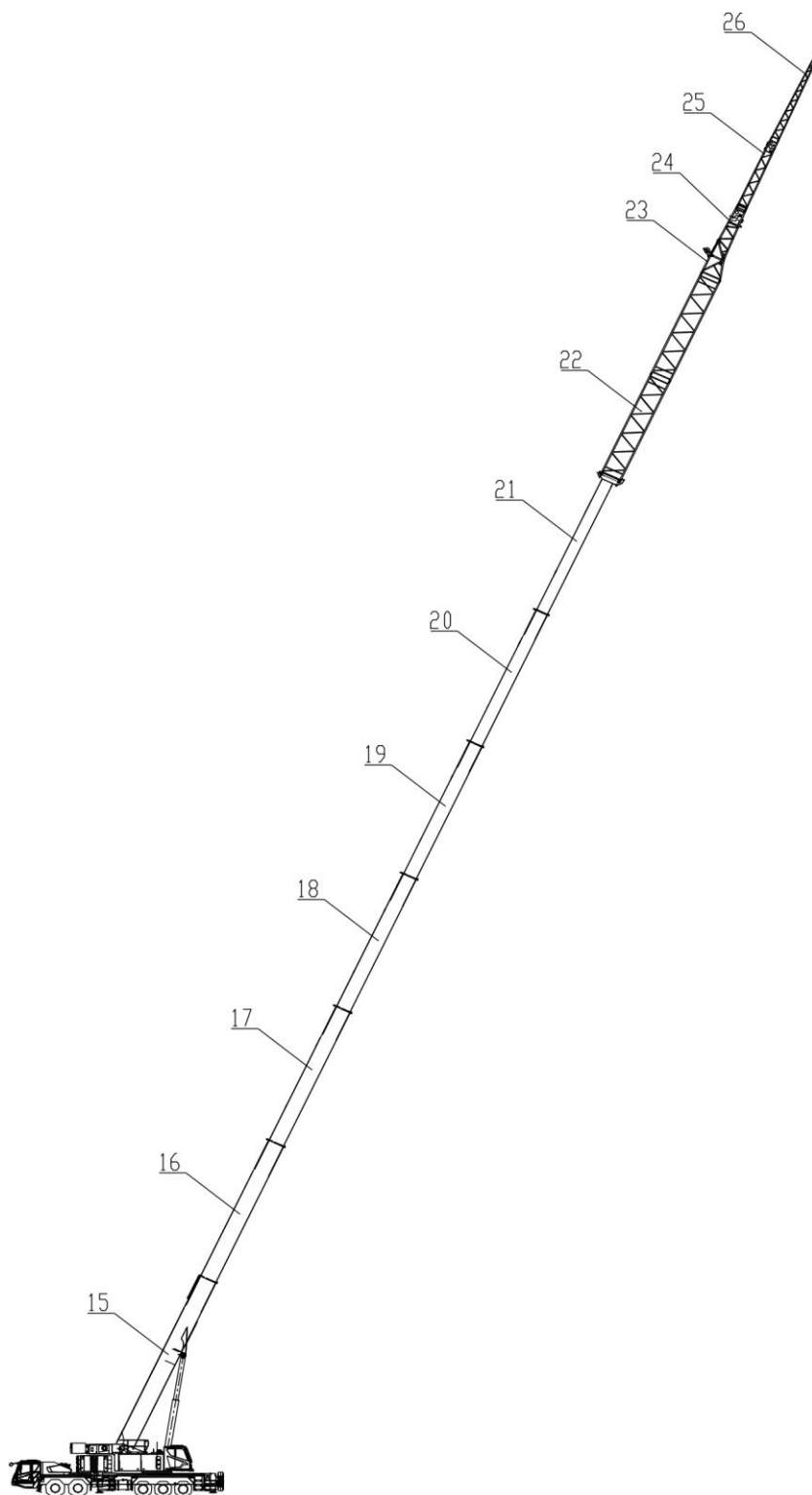
Figura 1-6 Principais Componentes do Produto (continuação)
