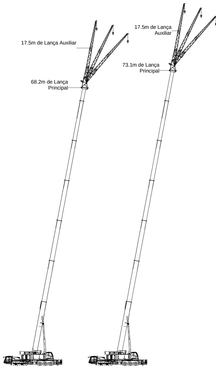
Figura 1-9 Lança Principal + +17,5m de Lança Auxiliar
