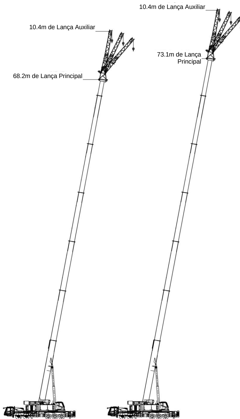
Figura 1-8 Lança Principal + 10,4m de Lança Auxiliar
