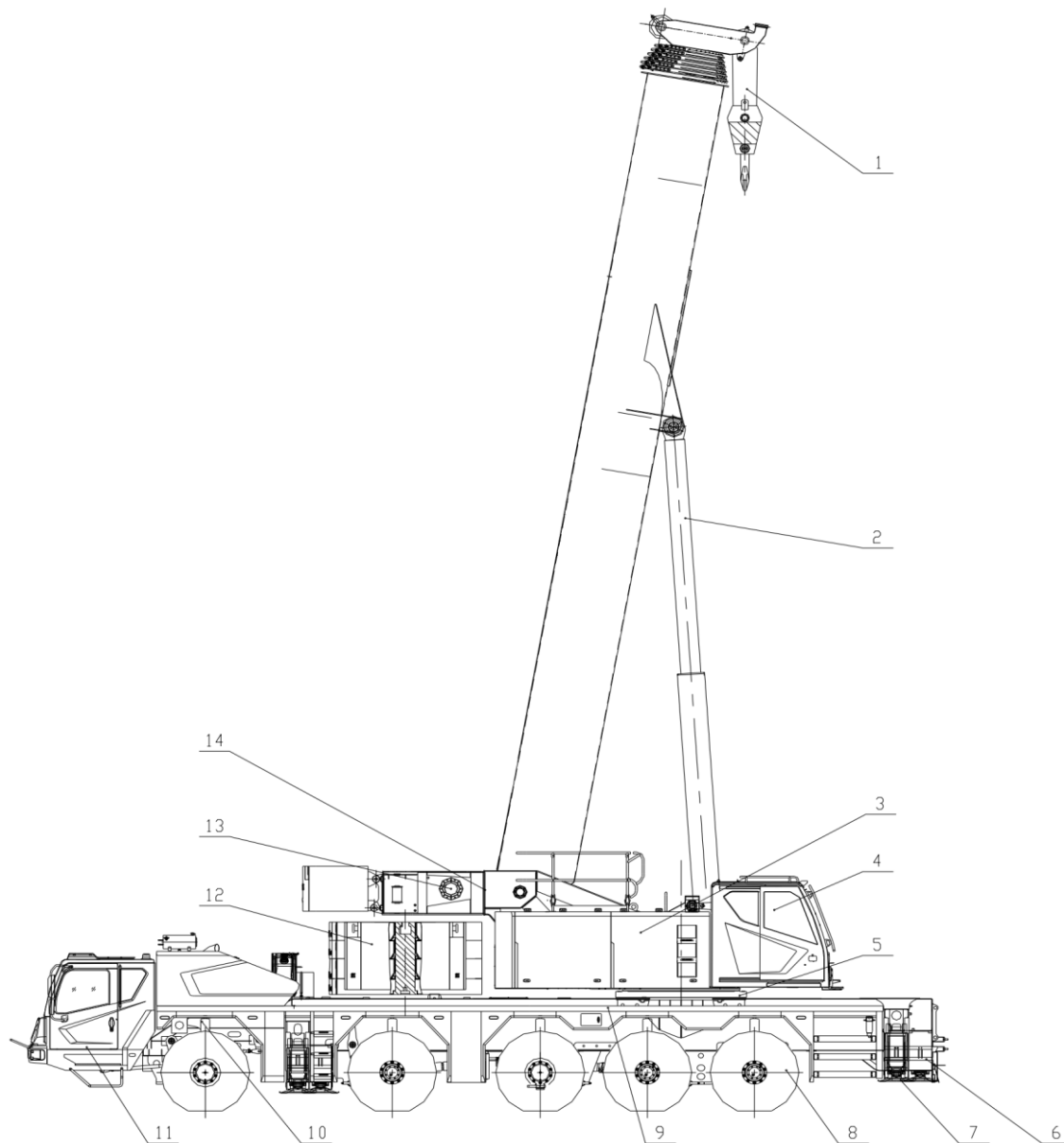
Figura 1-6 Componentes Principais do Produto
