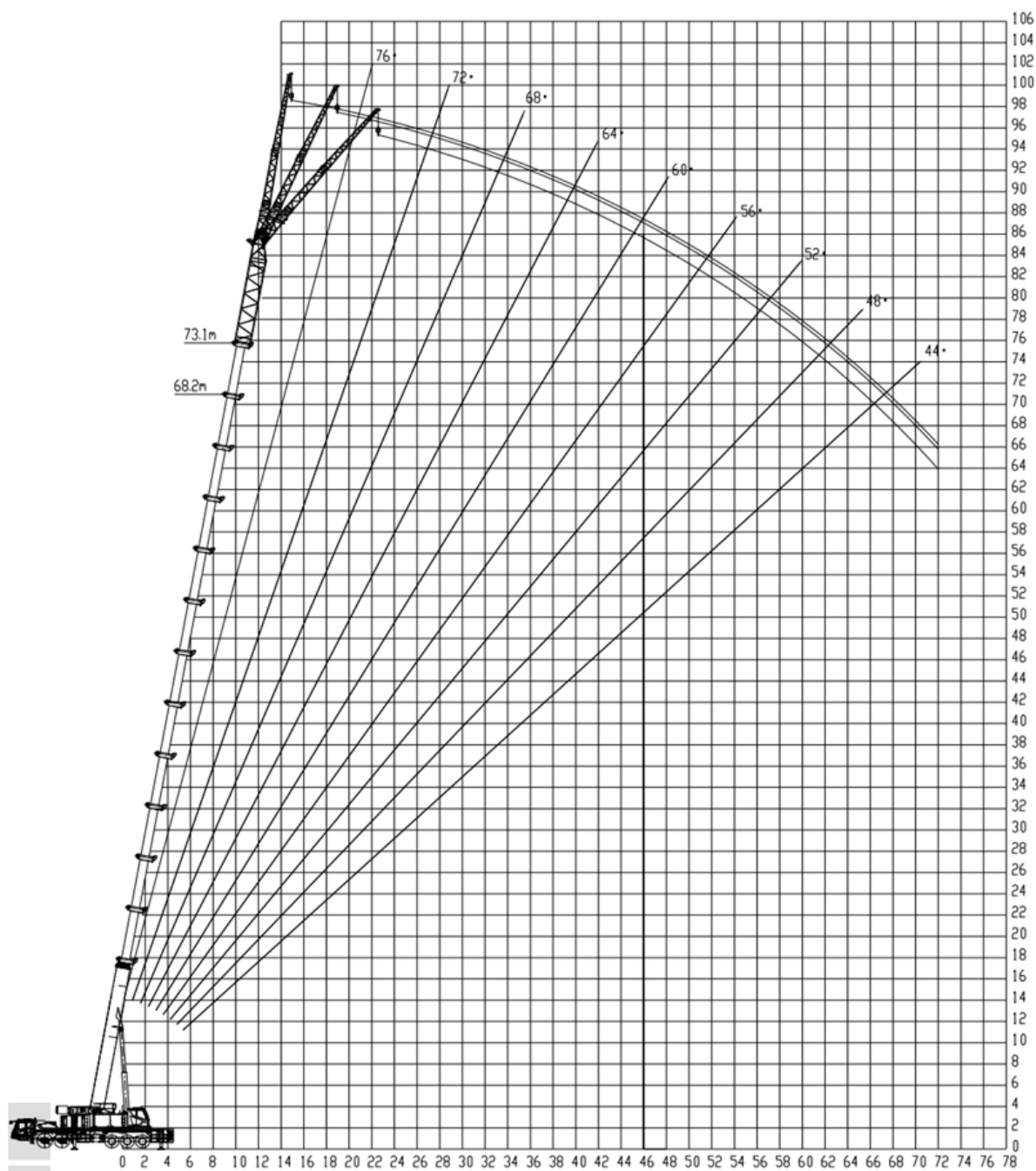
Figura 1-18 Curva de altura de elevação da lança principal + seção padrão de 8m + lança auxiliar de 17,5m
