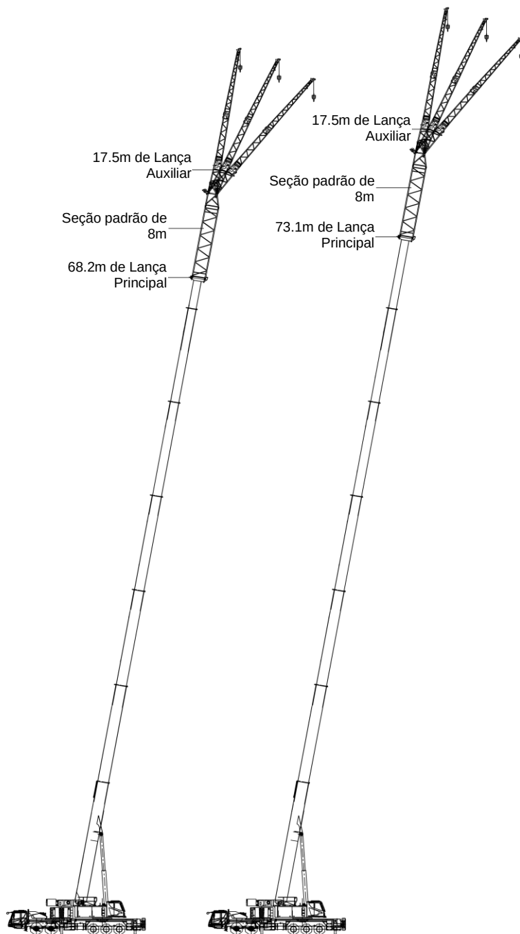
Figura 1-10 Lança Principal + +25,5m de Lança Auxiliar
