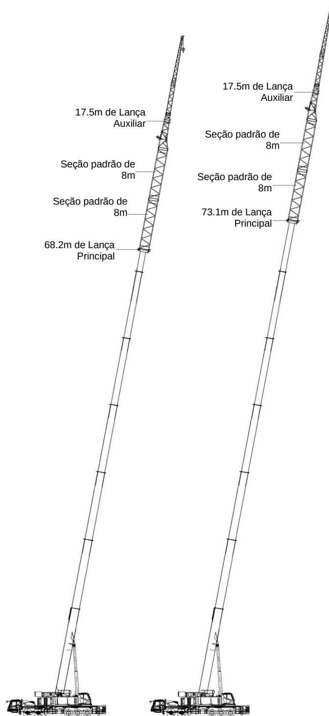
Figura 1-11 Lança Principal + +33,5m de Lança Auxiliar
