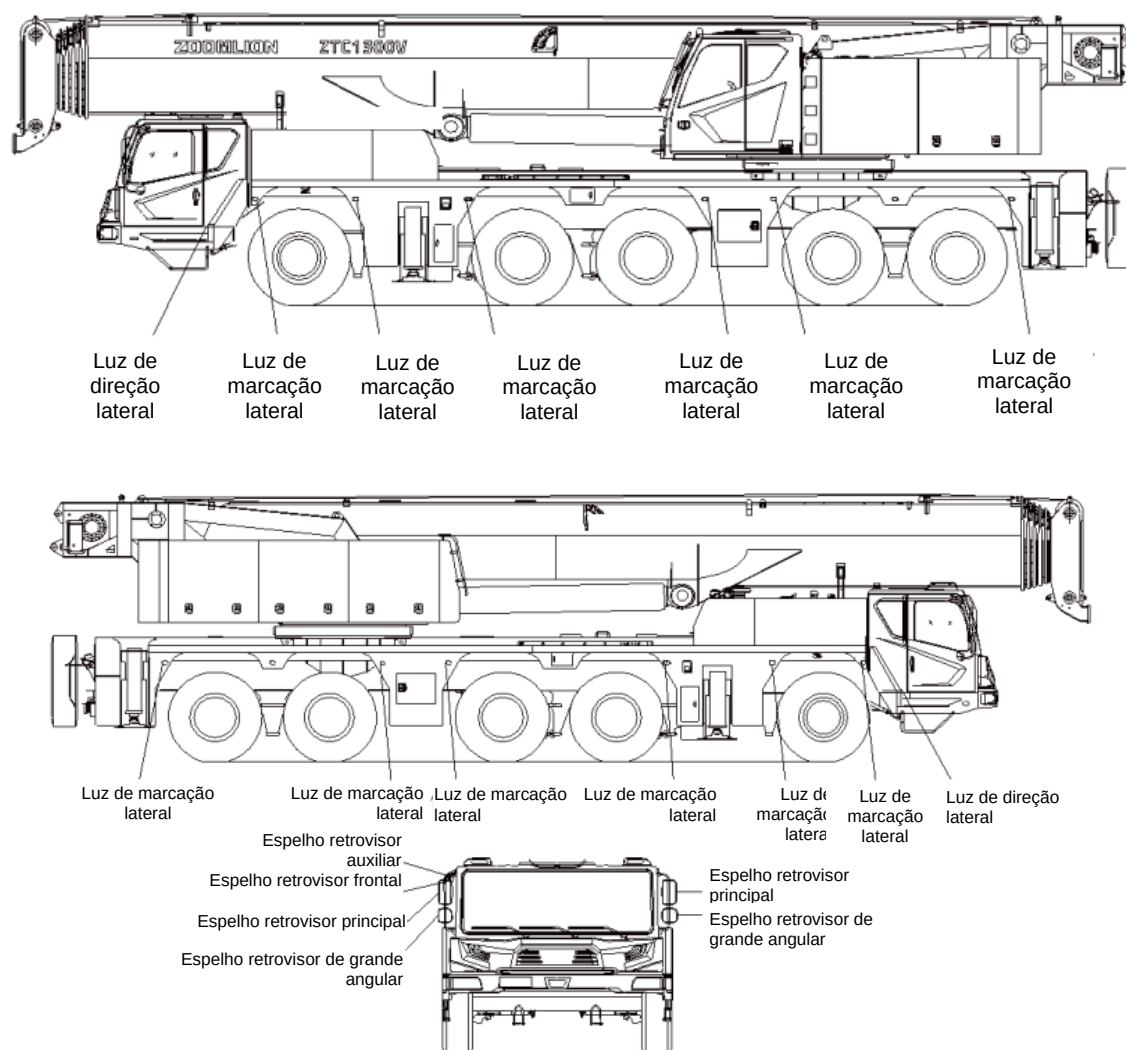
Figura 1-26 Nome e localização dos componentes não considerados nas dimensões externas do veículo conforme a norma GB1589
