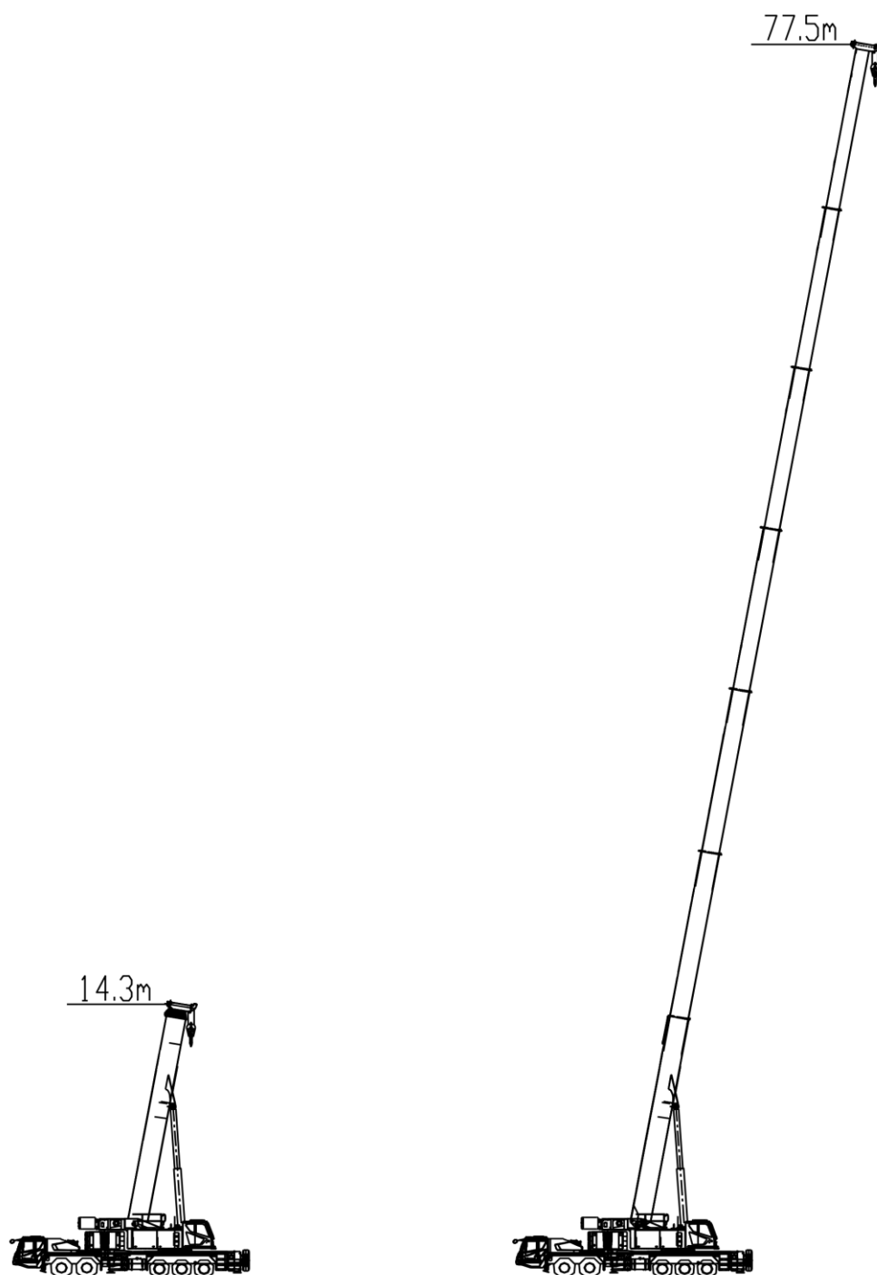
Figura 1-7 Lança Principal
