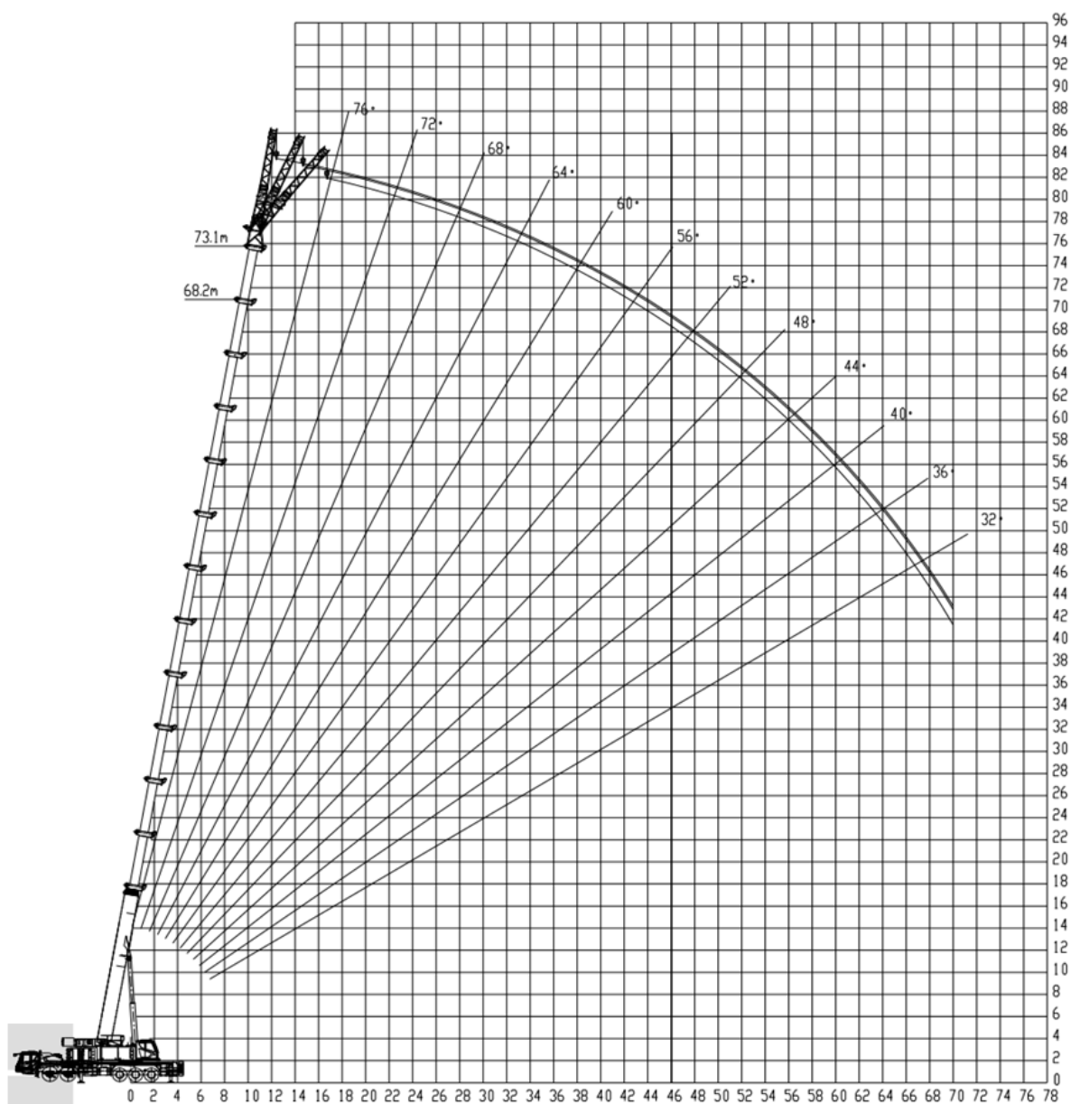
Figura 1-16 Curva de altura de elevação da lança principal + lança auxiliar de +10,4m
