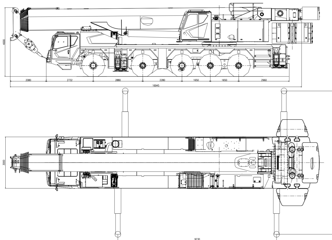
Figura 1-13 Parâmetros de Dimensões Externas
