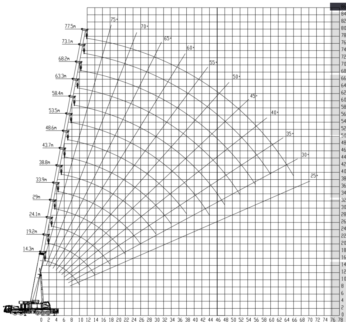
Figura 1-15 Curva de altura de elevação da lança principal
