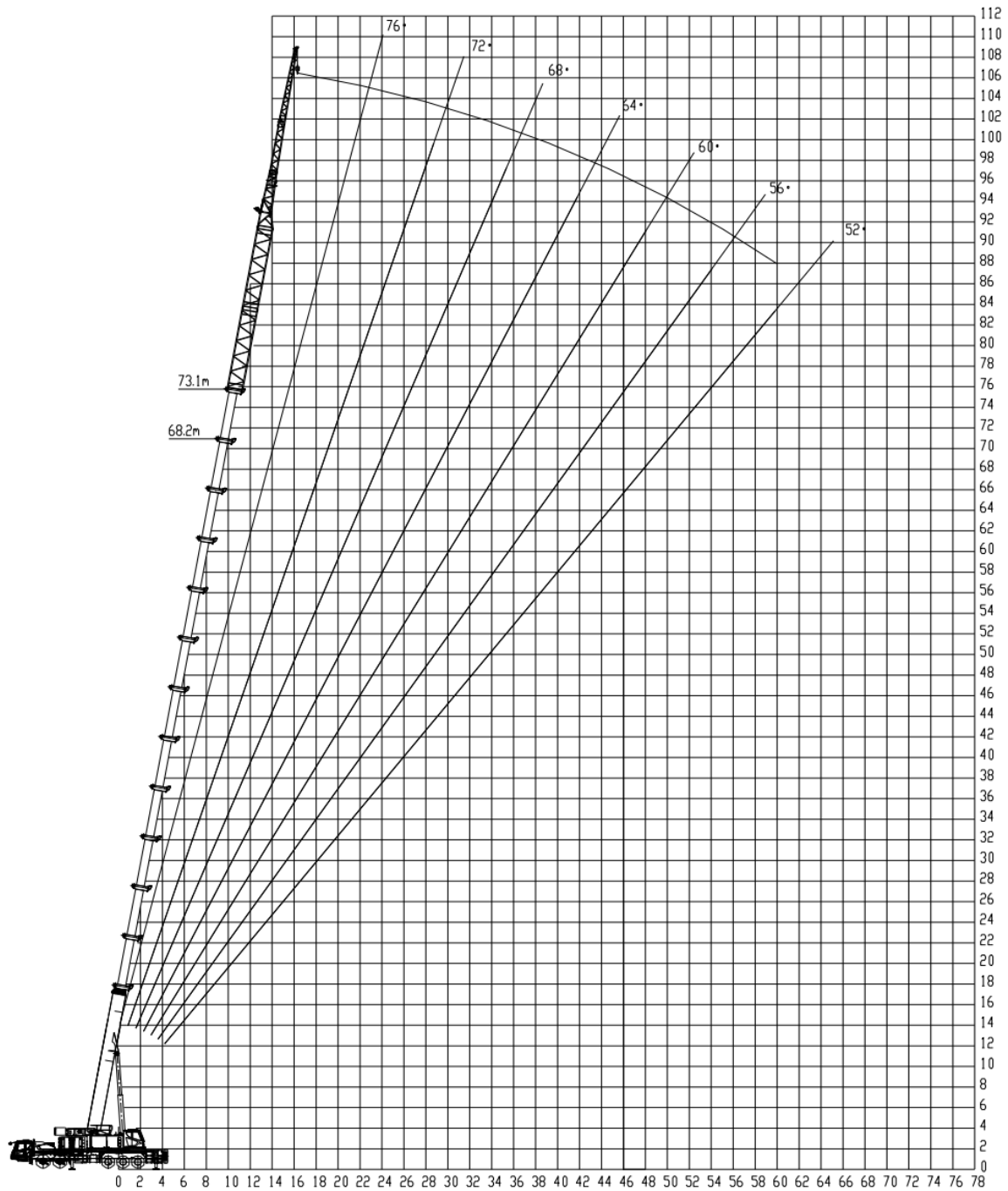
Figura 1-19 Curva de altura de elevação da lança principal + seção padrão de 8m + seção padrão de 8m + lança auxiliar de 17,5m
