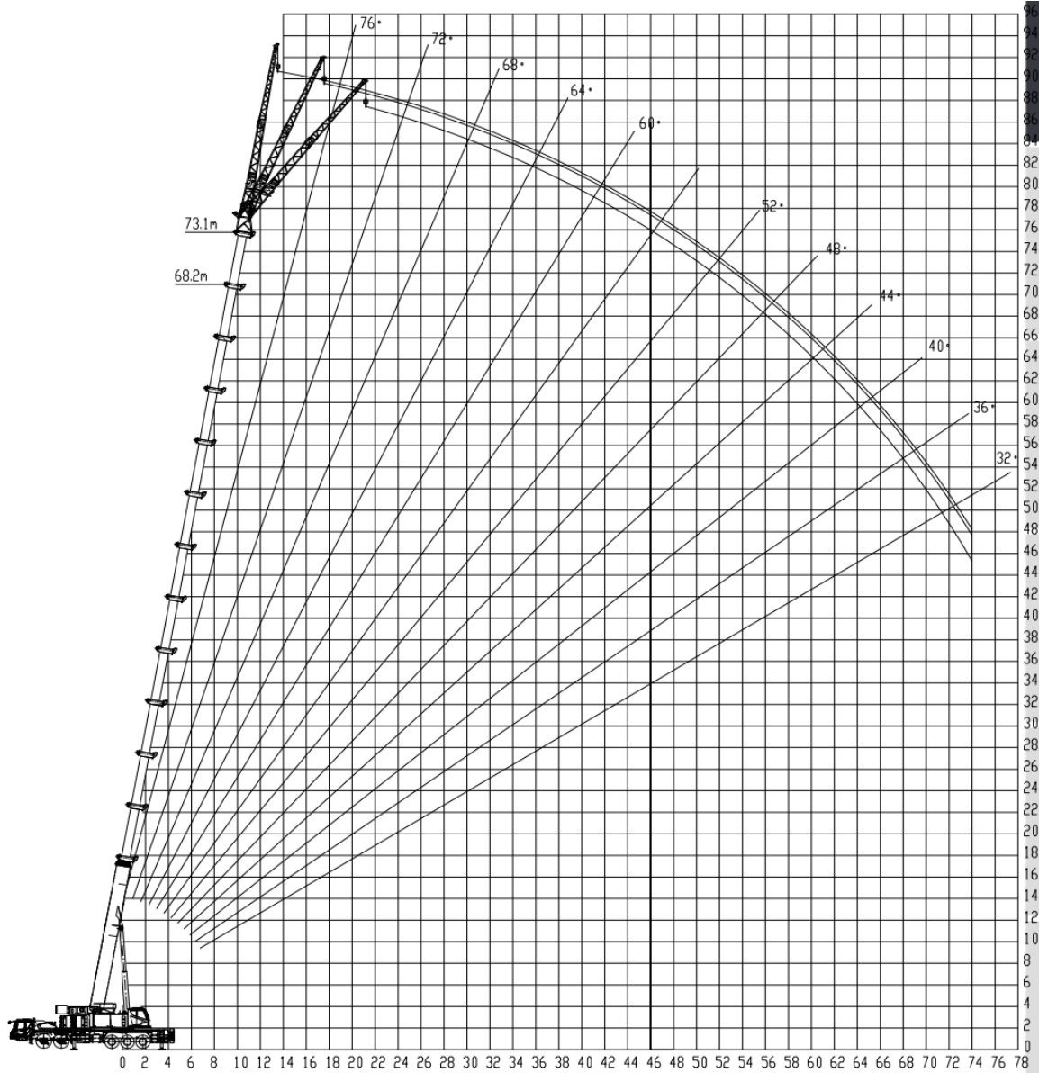
Figura 1-17 Curva de altura de elevação da lança principal + lança auxiliar de 17,5m
